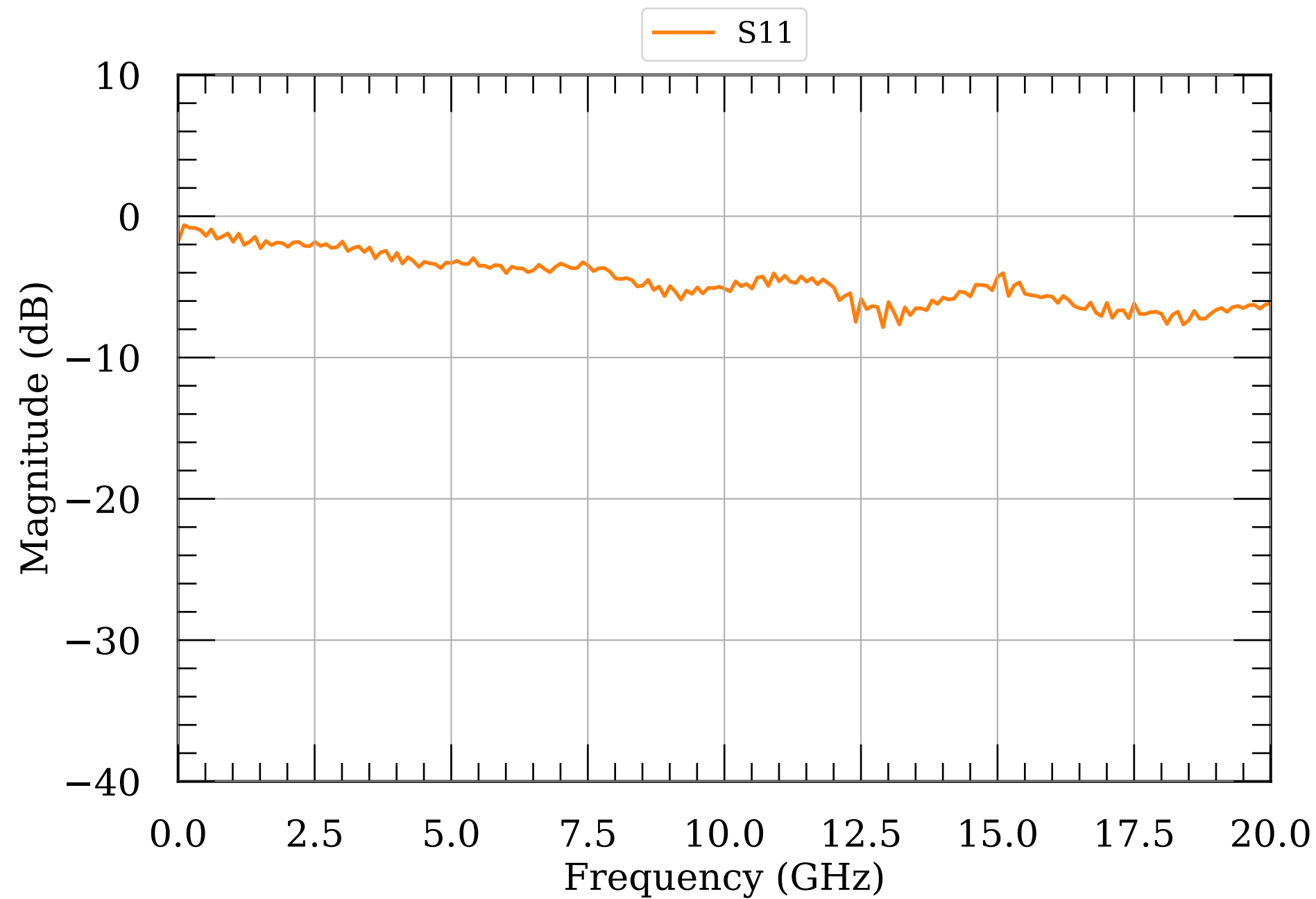
LNA S-params module053
